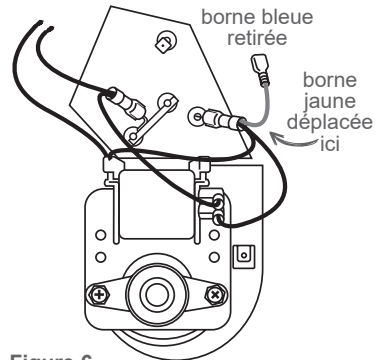
Figure 6 retirer la borne bleue et appliquer du ruban électrique à l'extrémité; fixer aux autres câbles à l'aide d'une attache mono-usage. Déplacer la borne jaune et la fixer là où la borne bleue était fixée.
