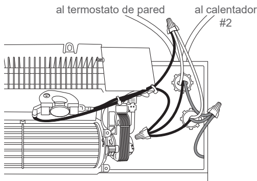
Figura 7 Calentador #1
