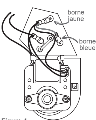
Figure 4 Astuce : Pour retirer les bornes plus facilement, tirer et remuer vers l'avant et l'arrière en même temps.
