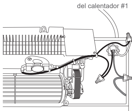
Figura 8 Calentador #2
