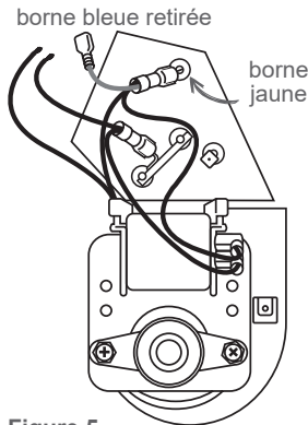
Figure 5 retirer la borne bleue et appliquer du ruban électrique à l'extrémité; fixer aux autres câbles à l'aide d'une attache mono-usage.
