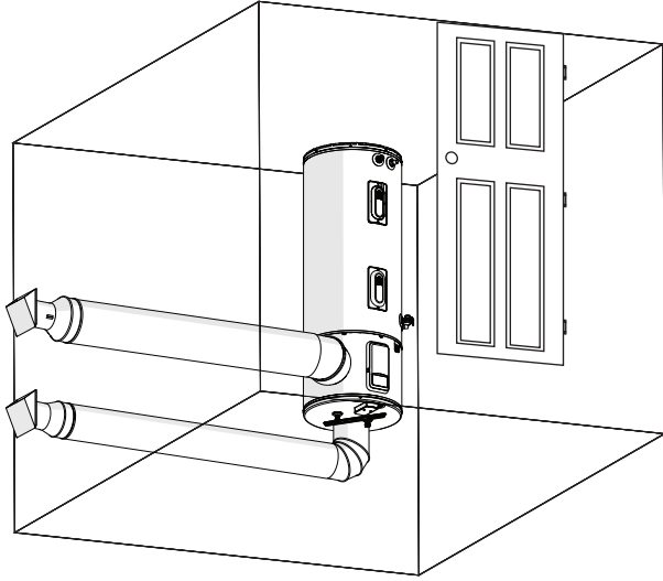
Chauffe-eau: avec conduit d'apport d'air ET d'évacuation
