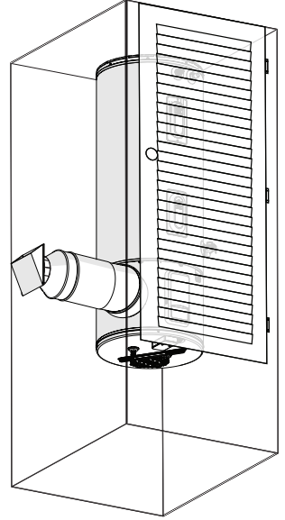
Chauffe-eau: avec conduit d'apport d'air OU d'évacuation
