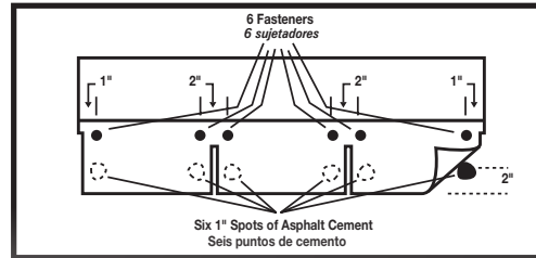
Fig. 3B Mansard or Steep Slope Pattern Esquema de mansarda o pendiente pronunciada
