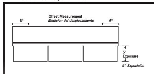
Fig. 4 Offset Measurement Medición del desplazamiento
