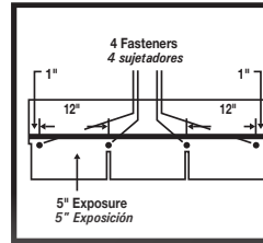
Fig. 3 Standard Pattern Esquema estándar
