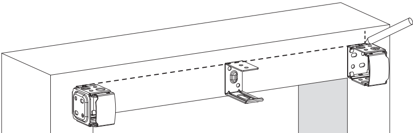
Supporting Bracket Soporte de apoyo
