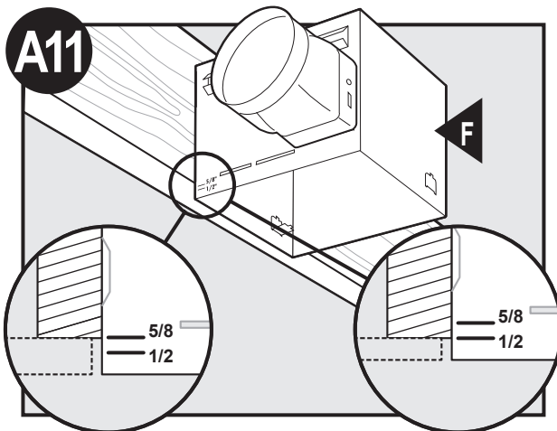
Ubique la marca de profundidad correcta en el borde inferior de la viga, según el espesor de su plancha de yeso.
