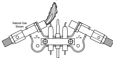
Figura 25 - Patrón incorrecto de la llama del piloto
