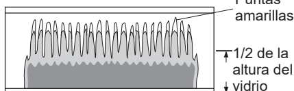
Figura 27 - Patrón incorrecto de la llama del quemador
