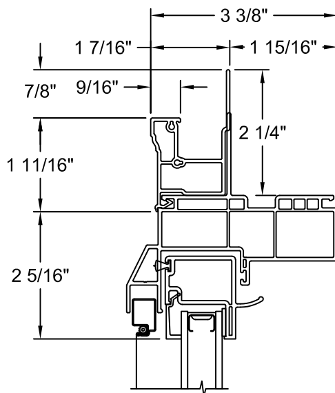
Brickmould
