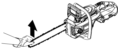
Fig. 32 LIFT THE TIP OF THE GUIDE BAR UP TO CHECK FOR SAG RELEVER L'EXTRÉMITÉ DU GUIDE POUR VÉRIFIER LE MOU LEVANTE LA PUNTA DE LA BARRA GUÍA PARA REVISAR LA HOLGURA DE LA CADENA
