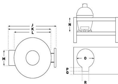
SEDD OVANIFRÅN
