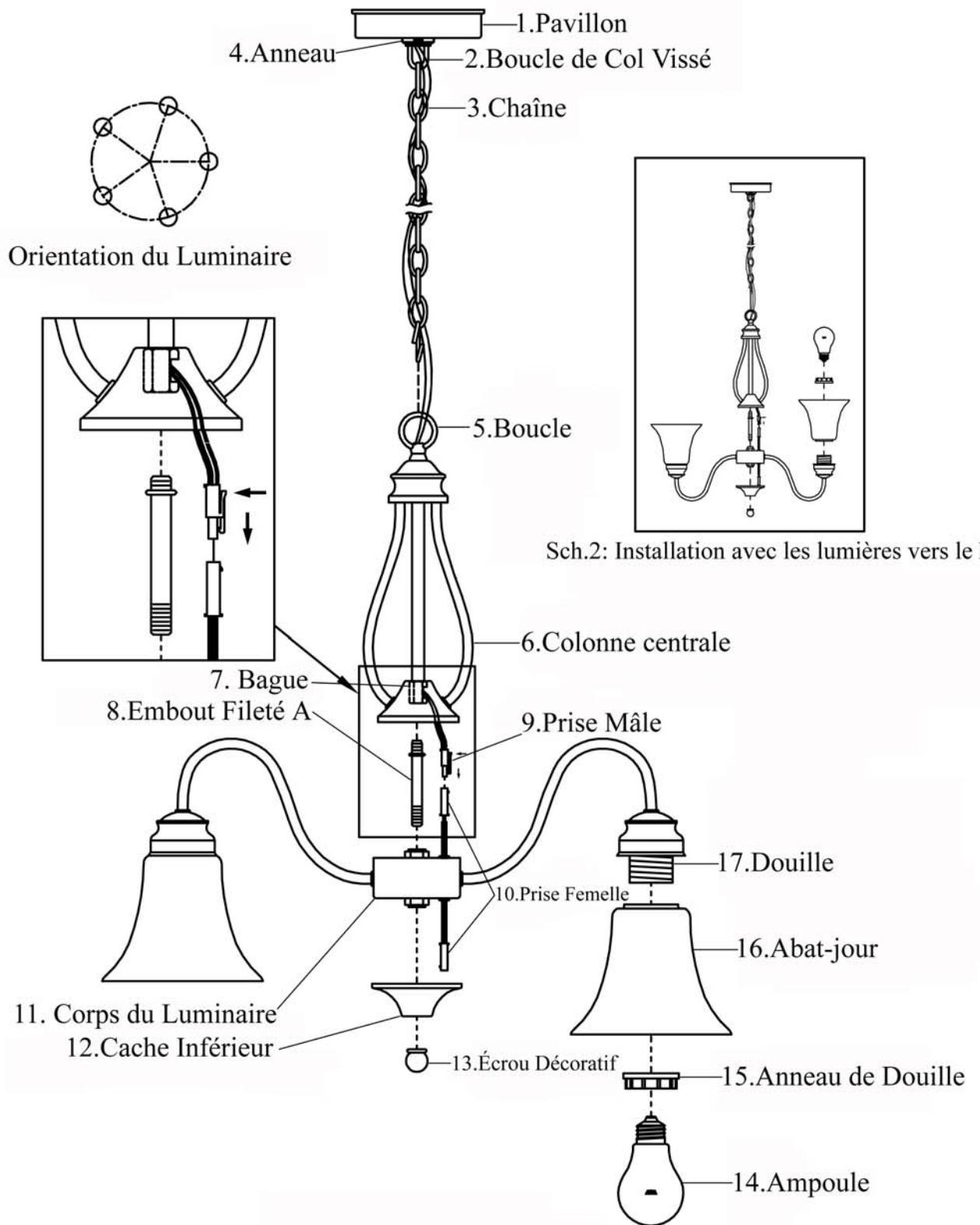
Sch.1 : Installation avec les lumières vers le bas
