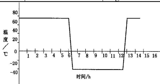
图 1 温度循环流程示意图
