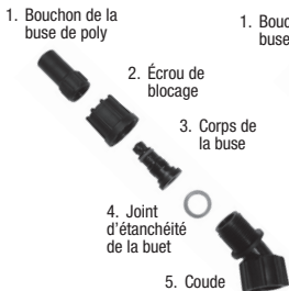
Figure 1 Buse ajustable en polyéthylène
