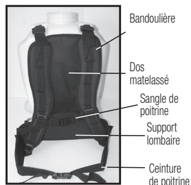
Figure 1 Assemblage de la sangle
