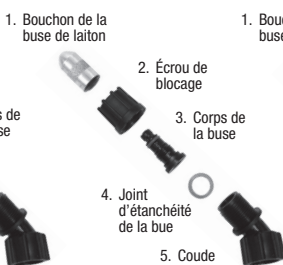
Figure 1 Buse ajustable en polyéthylène
