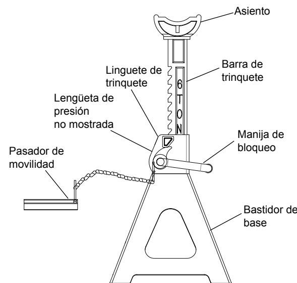
Figura 1: Nomenclatura habitual de un soporte de gato
