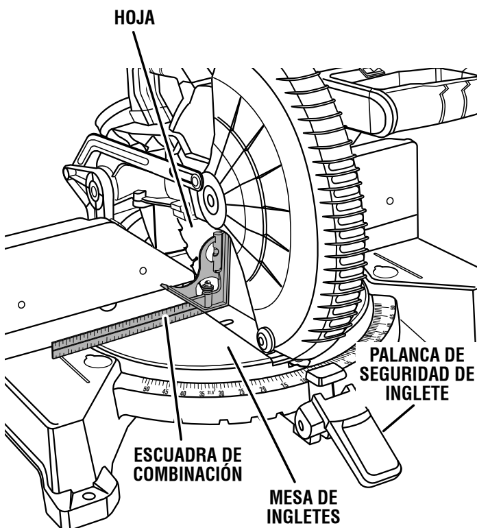
VISTA CORRECTA DE LA HOJA A ESCUADRA CON LA MESA DE INGLETES
