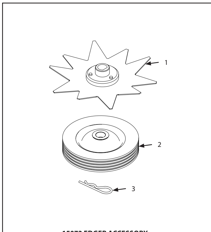
15073 EDGER ACCESSORY
