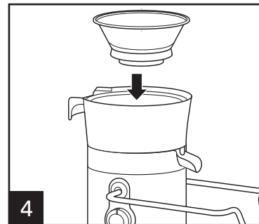
4 Placer le panier-filtre en acier inoxydable dans le bol de la centrifugeuse.
