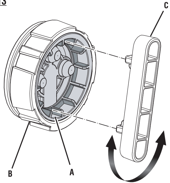
A - Threaded ring (anneau fileté, anillo roscado) B - Nozzle selector (sélecteur de buse, selector de boquilla) C - Nozzle tool (outil pour buse, herramienta para boquilla)
