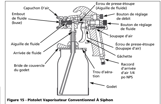
Figure 15 - Pistolet Vaporisateur Conventionnel À Siphon
