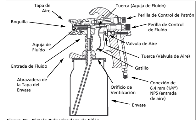
Figure 15 - Pistola Pulverizadora de Sifón
