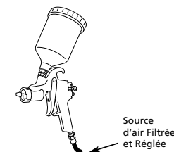
Figure 5 - Montage du Godet - Alimentation À Gravité
