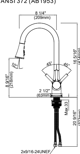
Diagramme schématique du produit
