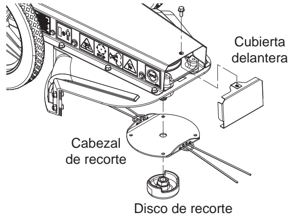
Figura 5.1, Regulación de altura de corte
