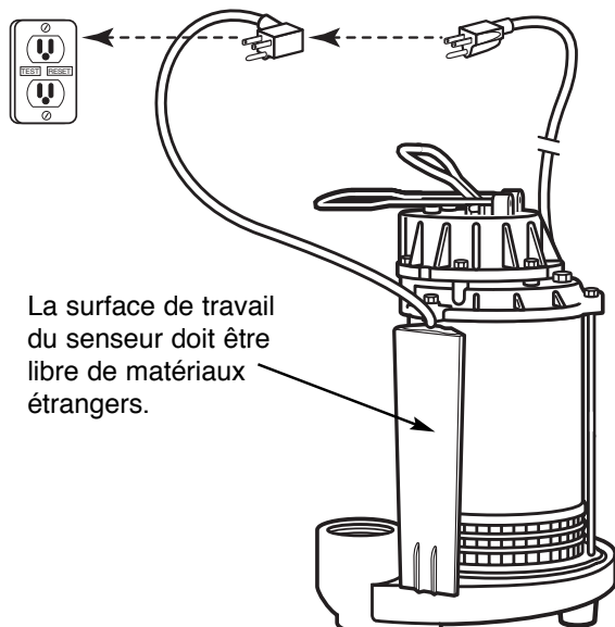
Figure 4 – Détecteur d'eau à état solide
