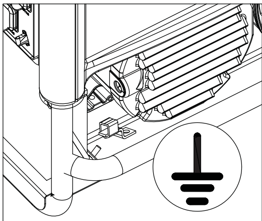
Figura 7 – Ubicación de la tierra del generador
