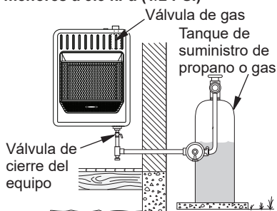
Figura 18 - Propano suministro de gas
