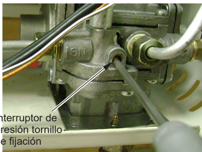
Figura 27 - Interrupción de presión del regulador de gas (Interior de la parte inferior del gabinete del calentador)
