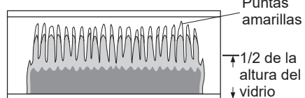
Figura 25 - Patrón incorrecto de la llama del quemador
