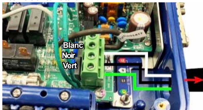
Boîtier de contrôle de 110 volts 30 ampères pour conversion sur le terrain
