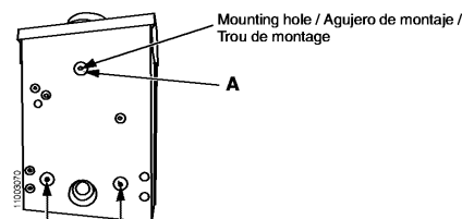
Mounting holes / Agujero de montaje / Trou de montage
