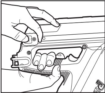
B. Appuyez sur le bouton et le suiveur se verrouillera en place.
