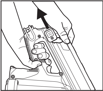
D. Tirer le suiveur jusqu'à la toute fin du guide, de sorte que le bouton sorte et que le suiveur se libère de cette position.
