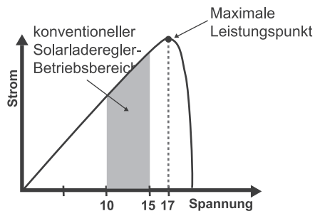
Ausgangsleistung (12V-System)
