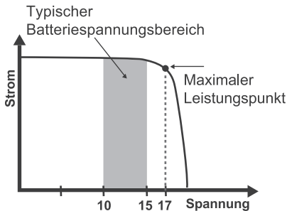
Strom und Spannung (12V-System)
