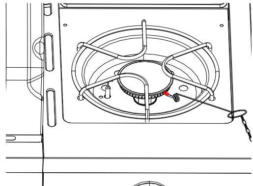
Allumage à l'allumette du brûleur latéral
