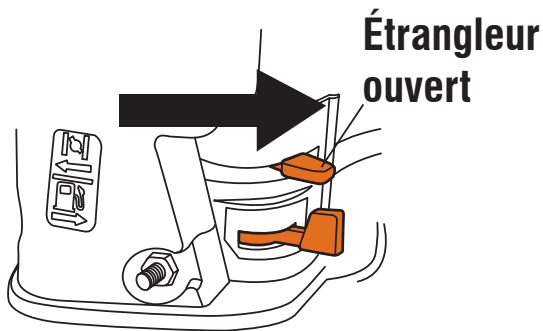
Figure 29 - Levier d'étrangleur
