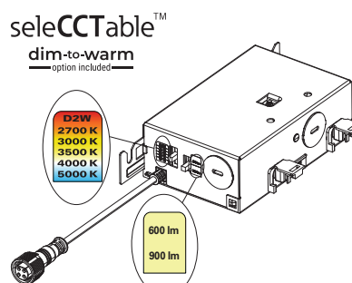
C. J-Box, CCT selectable & Lumen selectable Boîtier J, CCT sélectionnable & Lumen sélectionnable Caja de conexiones, CCT seleccionable y lumen seleccionable
