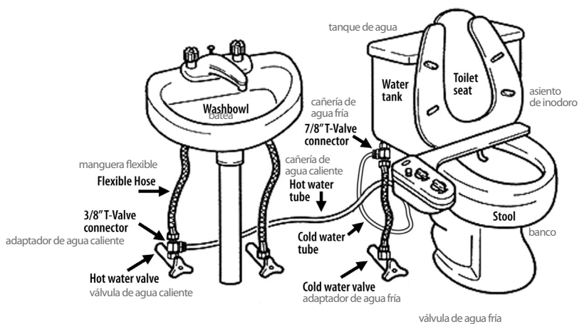
Vista de instalación completa con conexiones para agua CALIENTE y FRÍA
