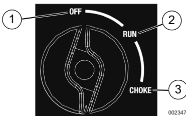
Figura 2-4. Interruptor (ejemplo)
