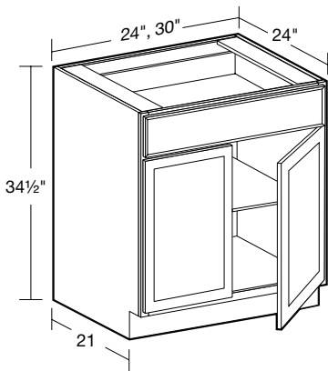
24" Deep Double Door
