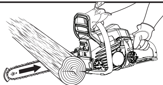
TRONZADO POR ABAJO Fig. 30
