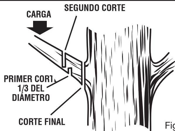
TRONZADO POR ABAJO Fig. 30
