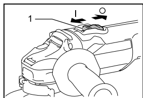
1. Interruptor deslizable
