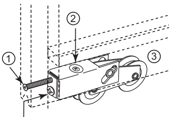
Adjustment screw Tornillo regulad Vis de réglage
