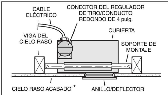
Instalación típica
