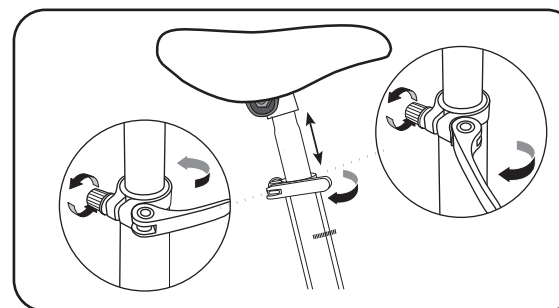
Système de fixation rapide de la selle
