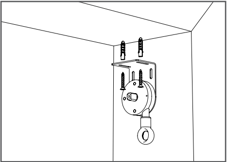
Montaje de soporte de molinete (B) en la parte superior. (Gire los tornillos 90° para montaje interno).
