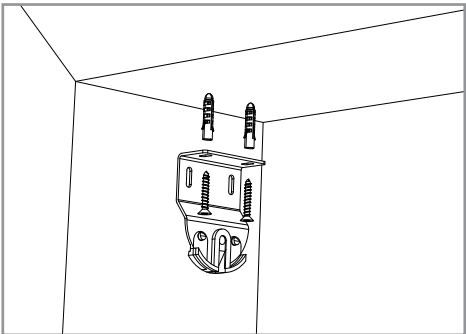
Montaje de soporte de molinete (A) en la parte superior. (Gire los tornillos 90° para montaje interno).
