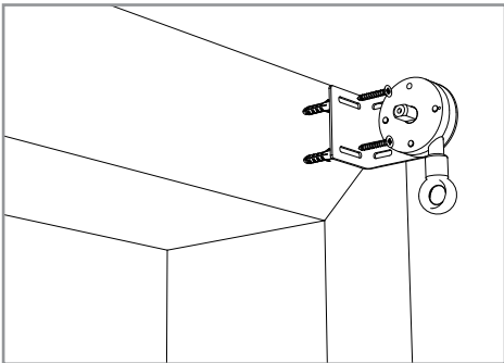
Soporte de polea para montaje exterior (B).
