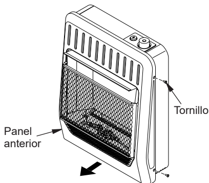
Figura 6 - Desmontaje del panel anterior
