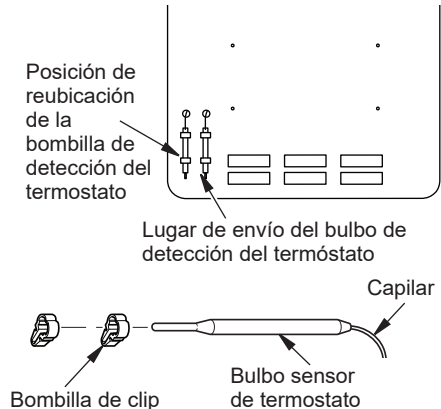
Figura 5 - Mover bulbo sensor de termostato
