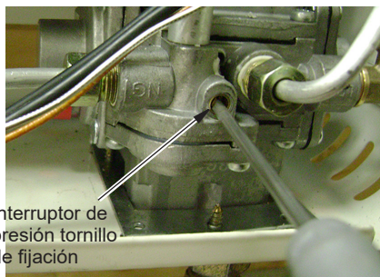
Figura 29 - Interruptor de presión del regulador de gas (Interior de la parte inferior del gabinete del calentador)
