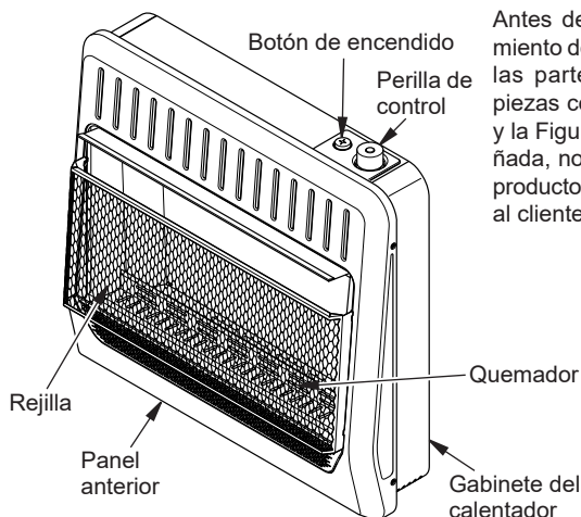
Figura 1 - Calentador de gas sin ventilación
