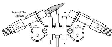
Figura 24 - Patrón correcto de la llama del piloto
