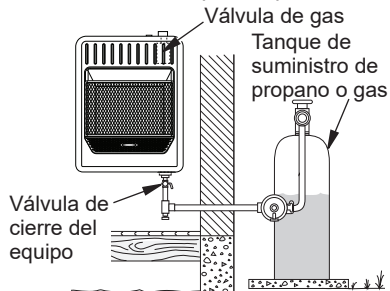
Figura 19 - Propano suministro de gas
