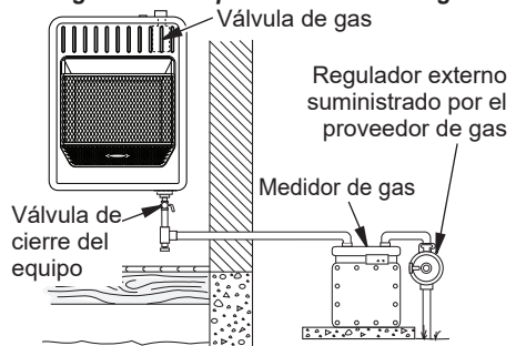
Figura 20 - Suministro de gas natural
