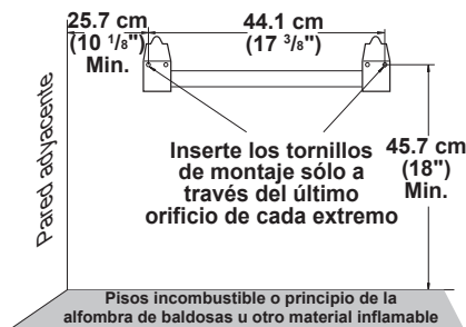
Figura 7 - Distancias mínimas del soporte de montaje
