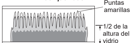
Figura 27 - Patrón incorrecto de la flama del quemador
