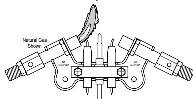
Figura 25 - Patrón incorrecto de la llama del piloto
