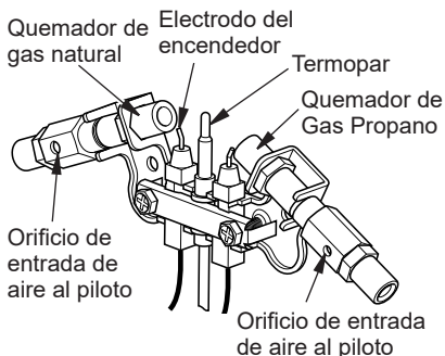
Figura 28 - Orificio de entrada de aire al piloto
