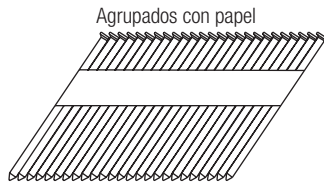
Clavos con cabeza D para enmarcado, enganchados a 34° (agrupados con papel)
