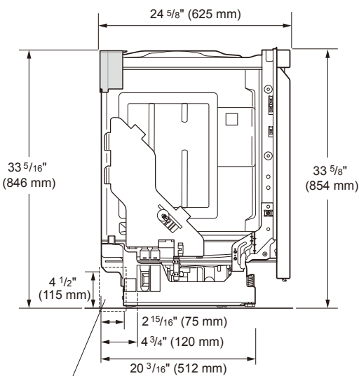
Vue latérale
