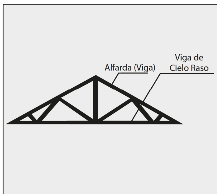
Fig.3. Estructura de Techo tipo Celosía.
