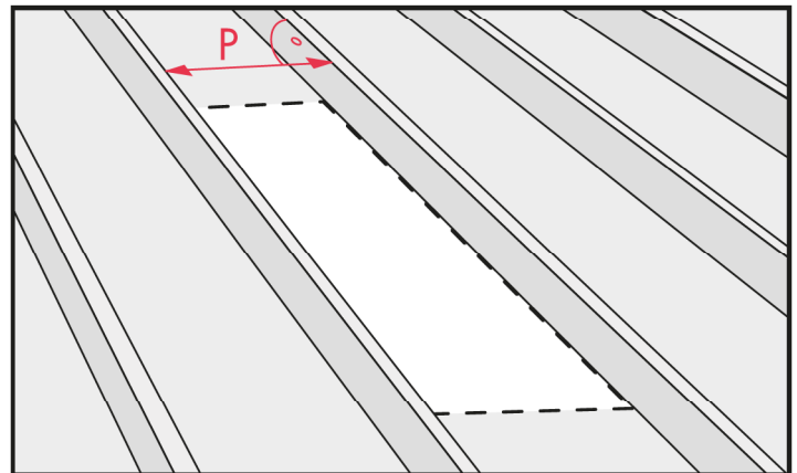
Fig. 12 P – Distance entre les solives de plafond.
