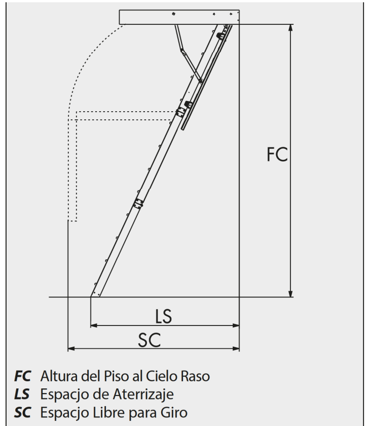
Fig.4. Características de una escalera de ático.
