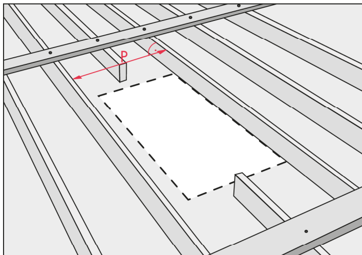
Fig. 15 P – Distance entre les solives de plafond.
