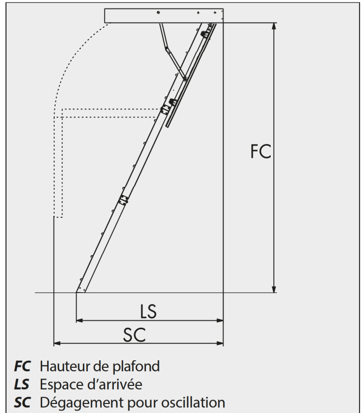
Fig. 4 Dimensions caractéristiques d'escalier.
