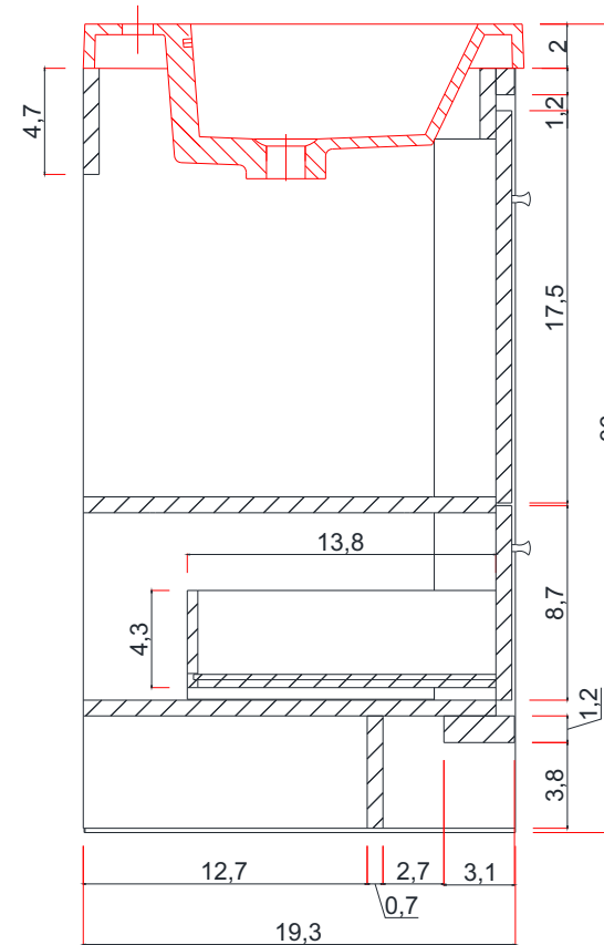
A-A KESİTİ
