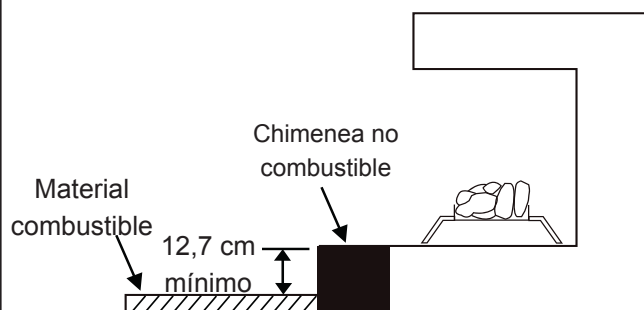
Fig. 8: Distancias de separación mínimas de la chimenea sobre los pisos combustibles
