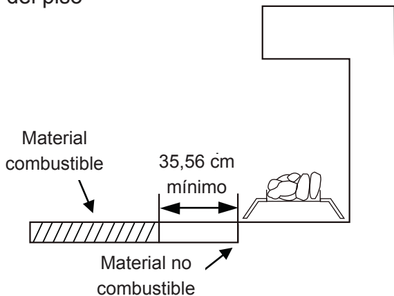
Fig. 7: Distancias de separación mínimas si la instalación es al nivel del piso
