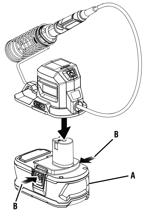
A - Battery pack (bloc-pile, paquete de baterías) B - Depress latches to release battery pack (appuyer sur les loquets pour retirer le bloc-piles, para soltar el paquete de baterías oprima los pestillos)
