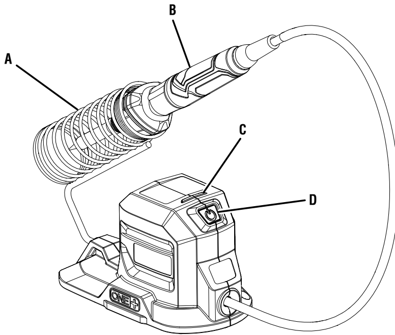
A - Pen holder (porte-stylo, soporte correspondiente) B - Soldering pen (stylo à souder, lápiz de soldador) C - LED indicator (témoin de DEL, luz indicadora de LED) D - On/off switch (commutateur marche/arrêt, interruptor de encendido/apagado)
