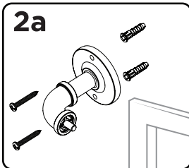
Wall mount installation for pipe brackets. Instalación de pared para soportes de tubo. Installation au mur des supports de tringle.
