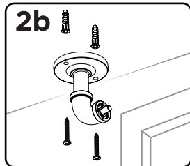
Ceiling mount installation for pipe brackets. Instalación de techo para soportes de tubo. Installation au plafond des supports de tringle.
