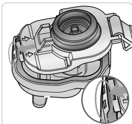
2. 스팀캡을 먼저 구멍에 맞춰 끼운 후 결합한다.
