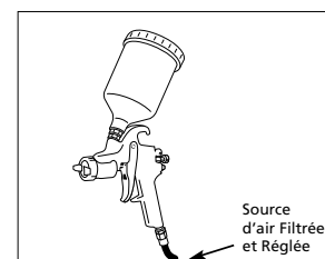
Figure 5 - Montage du Godet - Alimentation À Gravité
