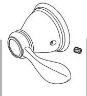
RP47842▲ Lever Handle w/Set Screw Palanca con Tornillo de Ajuste Manette avec vis de calage
